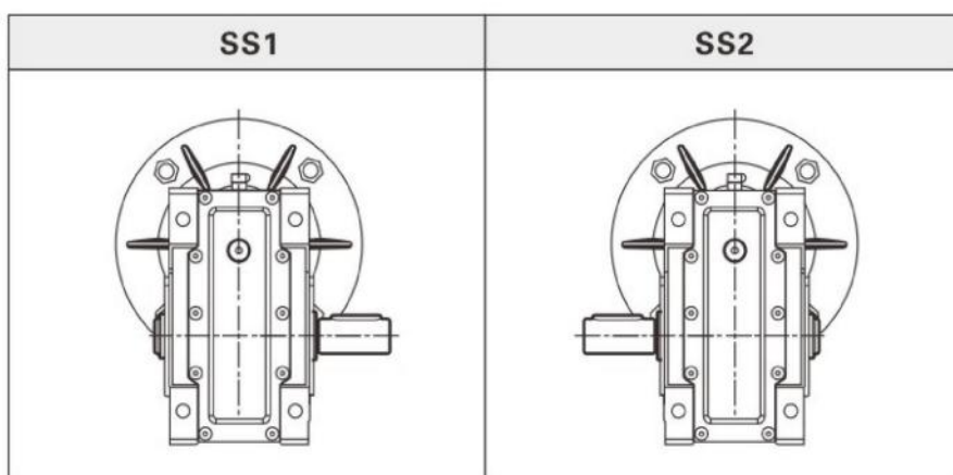
单向输出轴位置 / Position diagram for single output shaft
