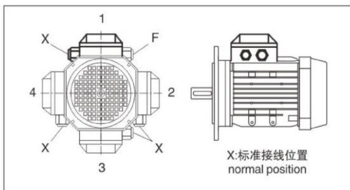
电机接线盒方位 / Position of motor terminal box
