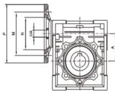
电机输入法兰 Motor input flange
