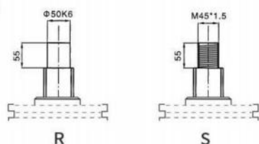
丝杆头部型式
