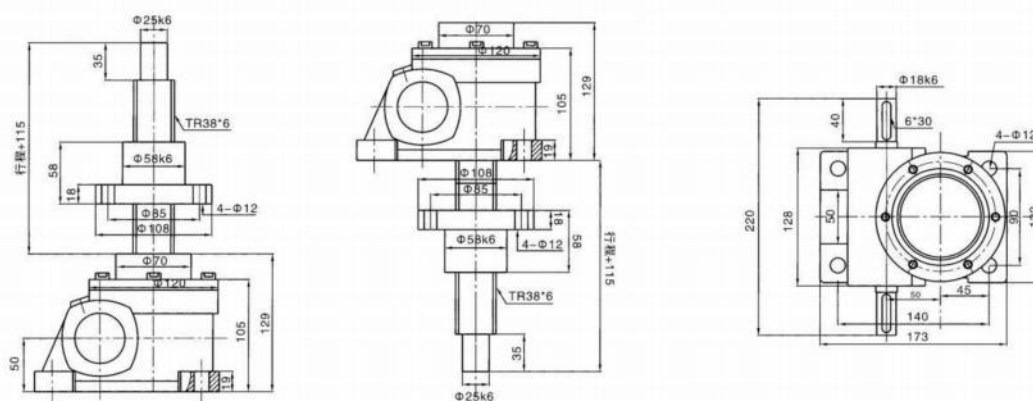
II 型结构型式
