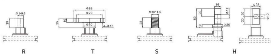
丝杆头部型式
