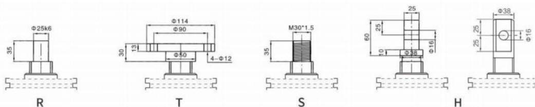
丝杆头部型式
