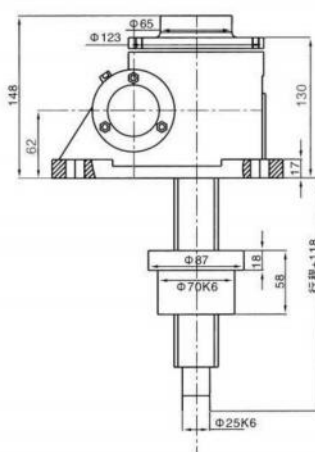
轴指向
