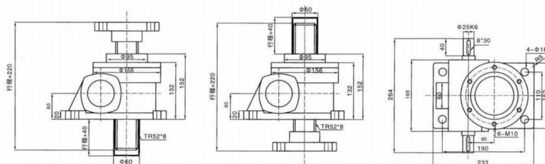
丝杆头部型式
