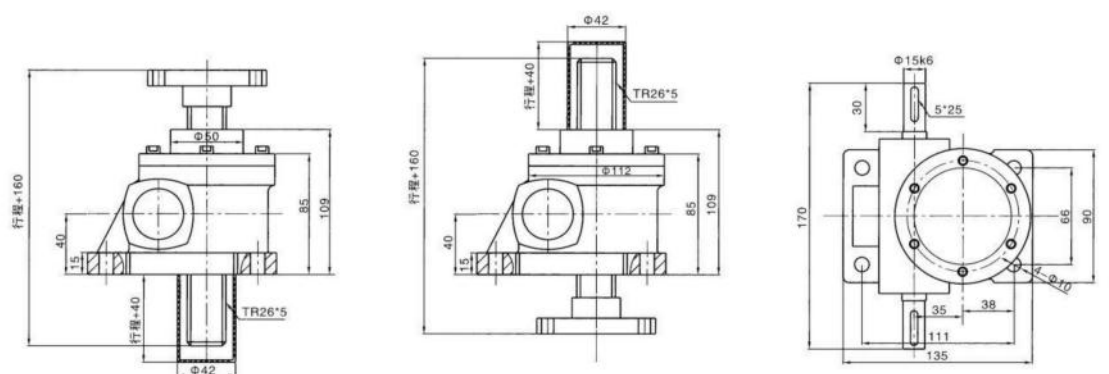
丝杆头部型式
