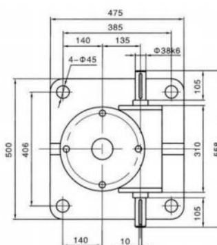
K向
