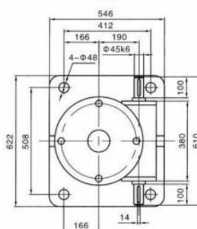
K向
