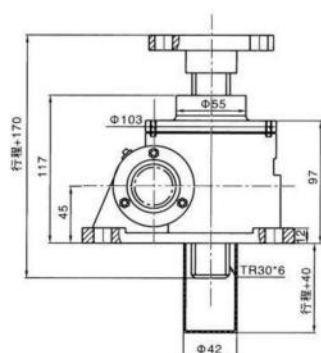
装配形式A
