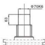
丝杆头部型式
