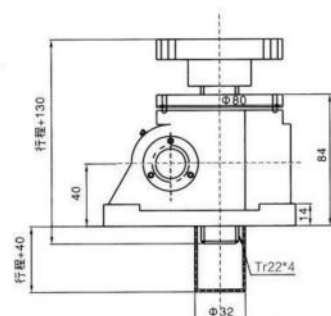
装配形式A
