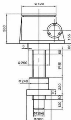
轴指向
