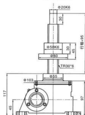
装配形式A
