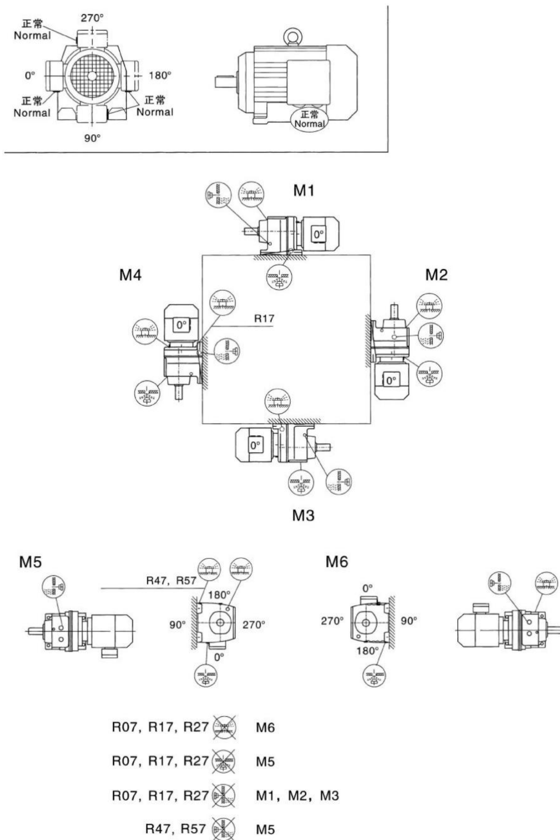
R07-R167安装形式图 R07-R167 Mounting position example
