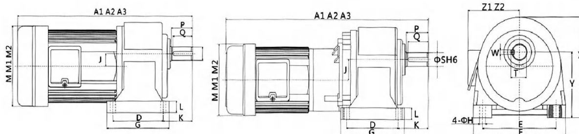
出力轴尺寸 output shaft
