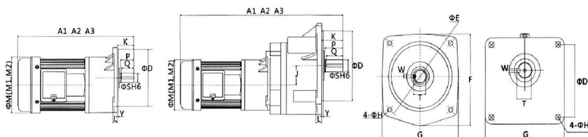
出力轴尺寸 output shaft
