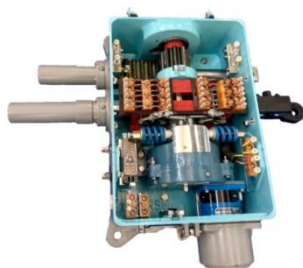
ZD6 系列电动转辙机 ZD6 Series Electric Switch Machine
