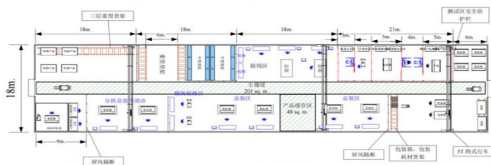
牵引系统检修新造车间布局规划图
