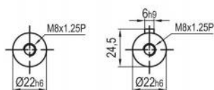
軸形式S1
