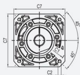
INPUT/輸入端
