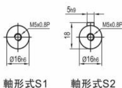
軸形式S1
