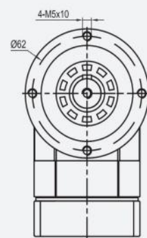
OUTPUT/輸出端
