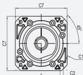
INPUT/輸入端
