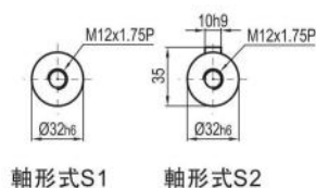
軸形式S1
