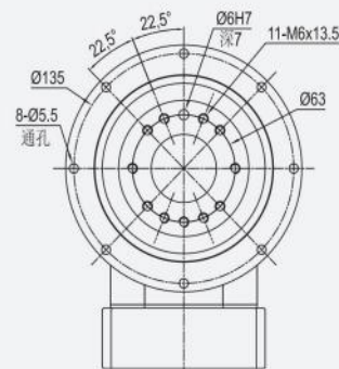
OUTPUT/輸出端
