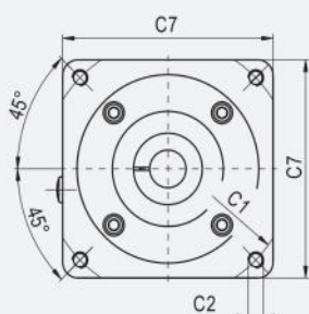
INPUT/輸入端
