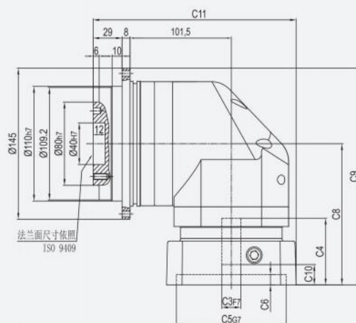
OUTPUT/輸出端
