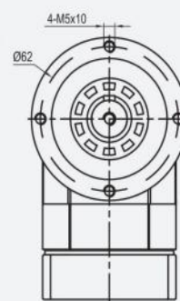
OUTPUT/輸出端
