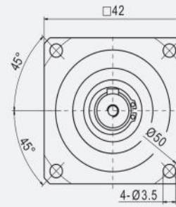
OUTPUT/輸出端
