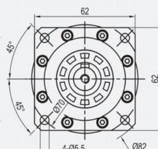
OUTPUT/輸出端
