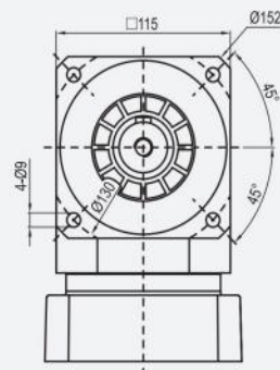
OUTPUT/輸出端
