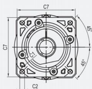
INPUT/輸入端
