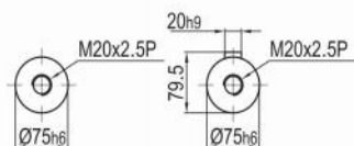
軸形式S1
