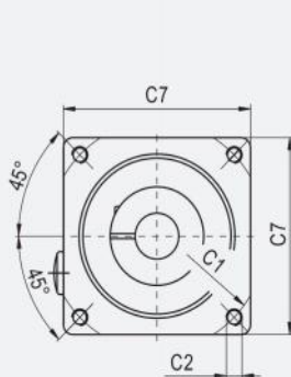
INPUT/輸入端
