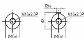
軸形式S1
