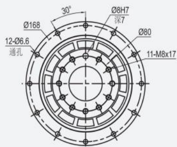
OUTPUT/輸出端
