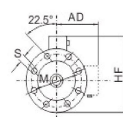
机座号(225-315) Frame size
