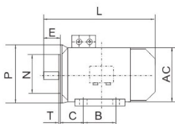
机座号(71-90) Frame size
