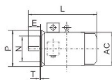
机座号(160-280) Frame size
