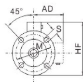
机座号(63-200) Frame size
