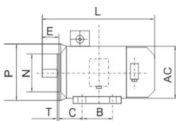
机座号(80-90) Frame size
