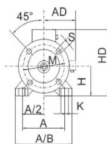
机座号(71-200) Frame size
