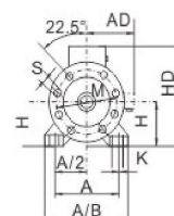
机座号(225-315) Frame size
