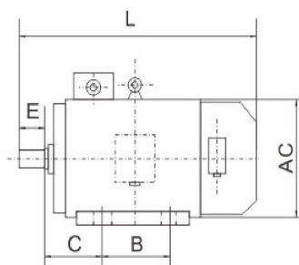
机座号(100-132) Frame size
