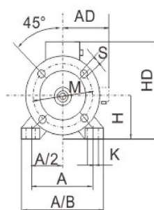
机座号(80-200) Frame size
