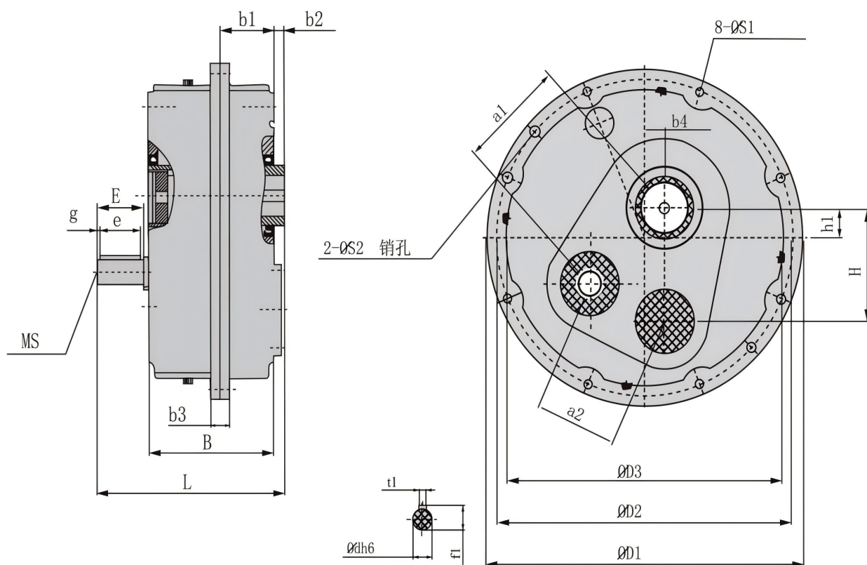
XG35-XG125的外形尺寸
